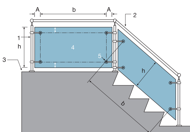
Figur 6a. Glas i rækværk fastholdt med gennemgående punktbeslag/bolte.
